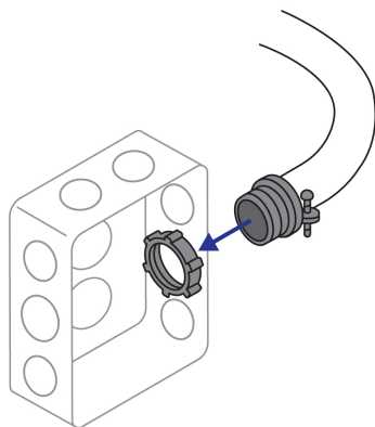
Ensamble de cable uso rudo a caja de registro
